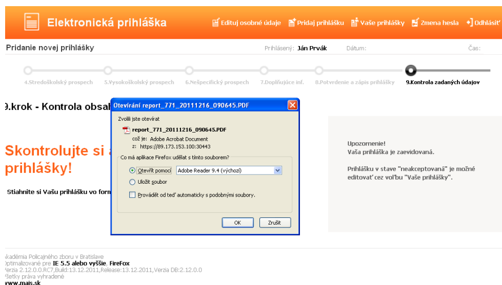
Obrázok 27 – Tlač prihlášky
